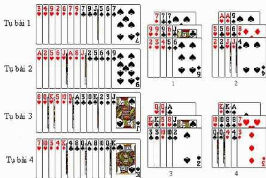
Ví dụ 1: Phân bố quân các tụ bài và cách Binh đúng đắn nhất.
