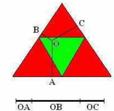
Hình 5: Minh họa bề que
