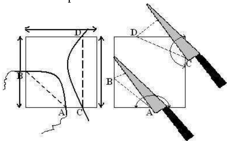
Hình 19: Cắt bằng lạt và bằng dao. Bánh để nguyên khi cắt xong đường cắt sau. Vết cắt thứ hai không được chồng lên vết đầu.
