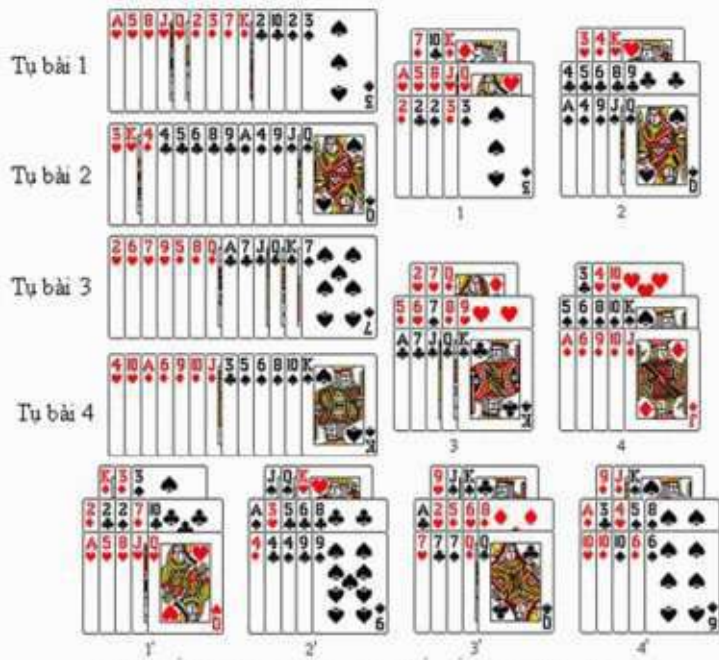
Ví dụ 2: Phân bổ quân các tự bài và cách Binh đúng đắn nhất.
