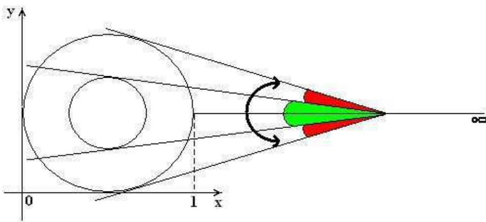
Hình 11: Nghịch lý Bertrand. Một điểm bên ngoài và thước kẻ.
