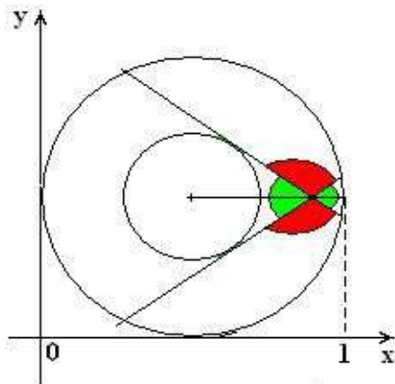
Hình 13: Nghịch lý Bertrand. Điểm bên trong và thước kẻ.
