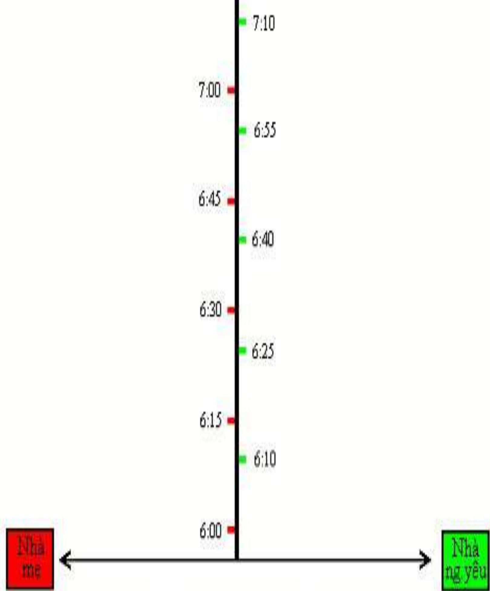
Hình 1: Lịch xe buýt tại điểm đợi của chàng trai về hướng mẹ ■ và người yêu □
