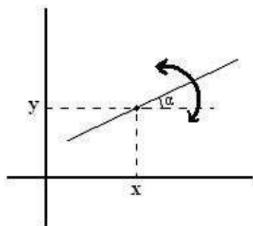
Cách 1: Điểm và thước kẻ
