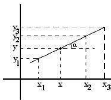
Cách 2: Nối hai điểm
