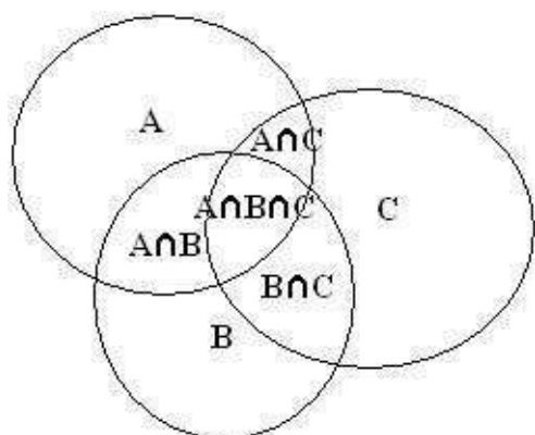
Hình 21: Biểu đồ Venn.
