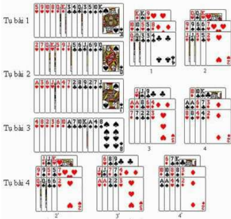
Ví dụ 2: Phân bổ quân các tu bài và cách Binh đúng đắn nhất. Cách 2', 3', 4' không theo logic thường nhưng hữu hiệu khi đã biết bài đối thủ.
