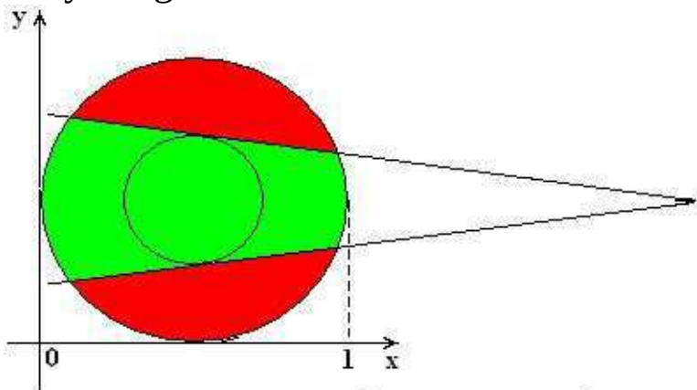
Hình 12: Nghịch lý Bertrand. Điểm bên ngoài và điểm bên trong.
