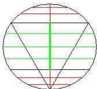
Hình 9: Nghịch lý Bertran 3
