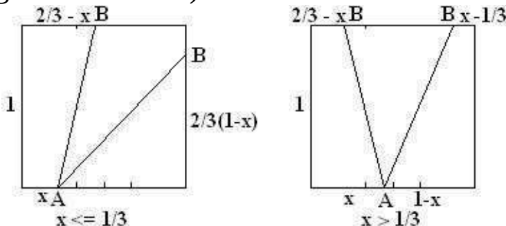
Hình 18: Trường hợp các điểm cắt ngẫu nhiên.
