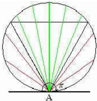
Hình 7: Nghịch lý Bertran 1
