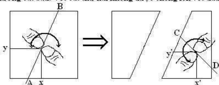
Hình 20: Bẻ. Bánh tách ra hai phần. Sau đó chọn một phần để bẻ tiếp. Điểm bẻ trong bánh và vết cắt ở bất kỳ đâu.
