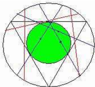
Hình 8: Nghịch lý Bertran 2
