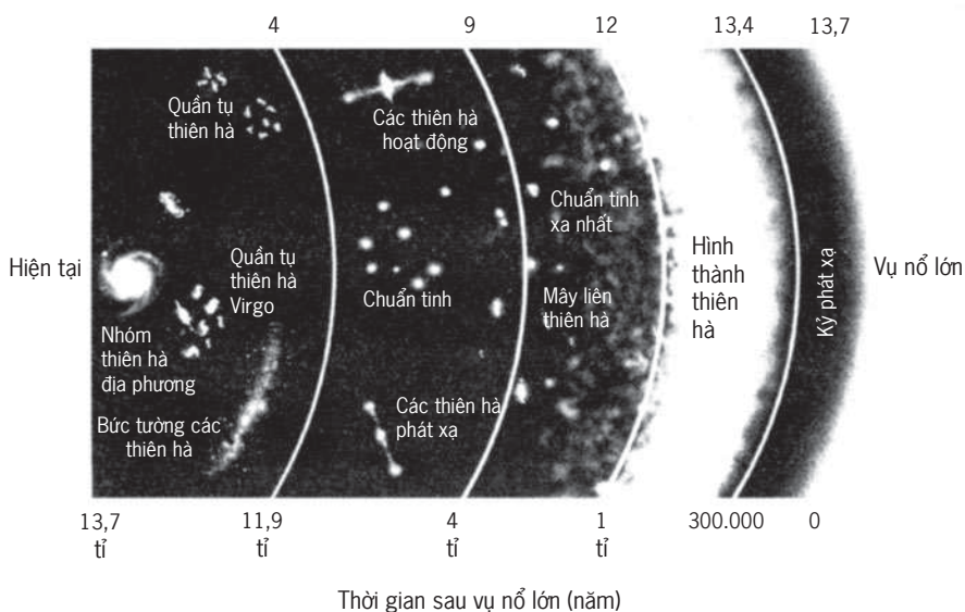
Hình 1.3 Vũ trụ như chúng ta thấy
