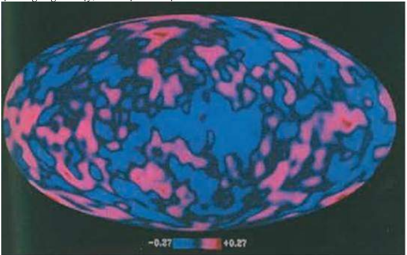
Bản đồ toàn bộ bầu trời do vệ tinh COBE chụp cho thấy các nếp nhăn theo thời gian.
