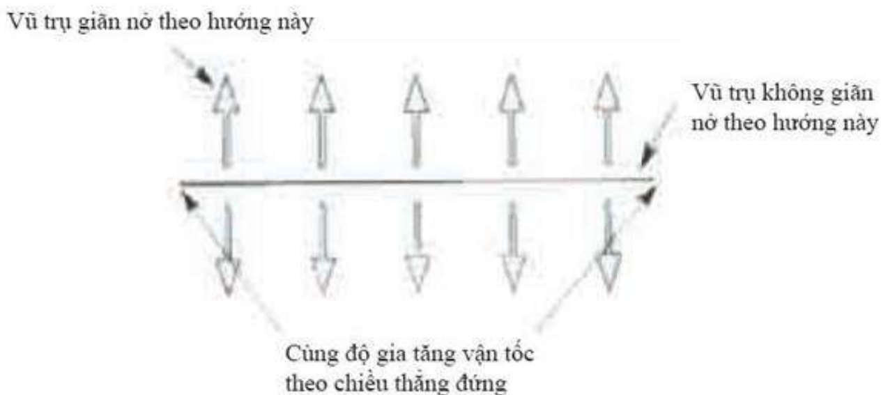
(Hình 5.18) VŨ TRỤ CÓ VÒNG THỜI GIAN ĐÓNG
