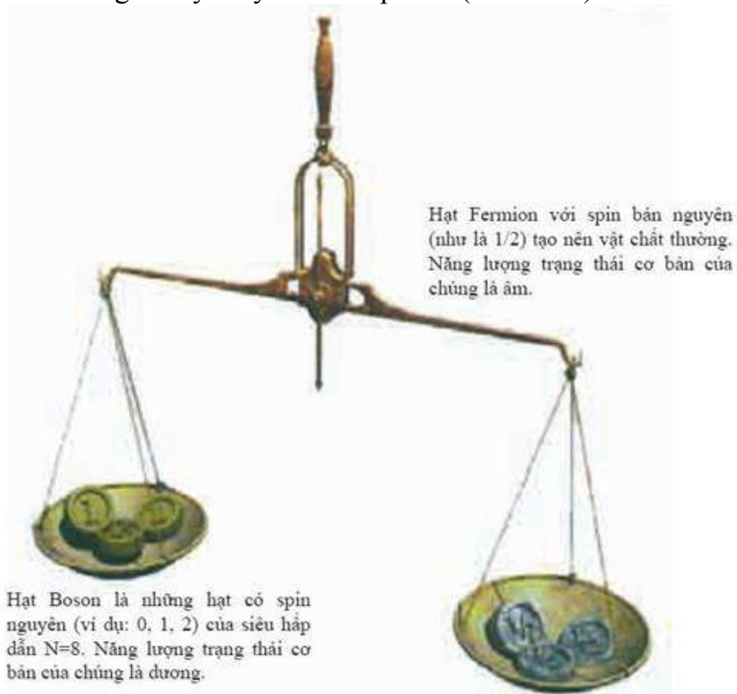
(Hình 2.13) SIÊU ĐỐI TÁC
