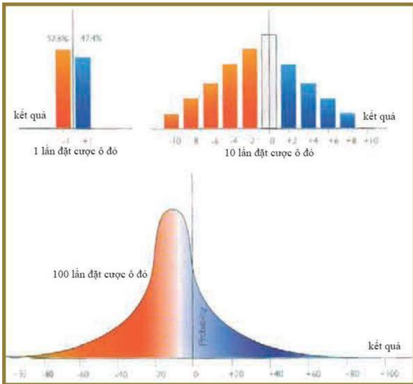
(Hình 3.7 và hình 3.8)
