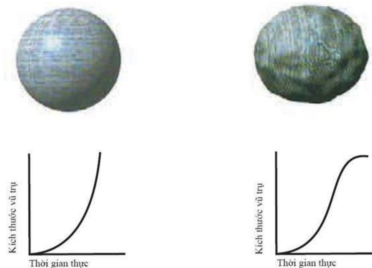
(Hình 3.15) VŨ TRỤ LẠM PHÁT
