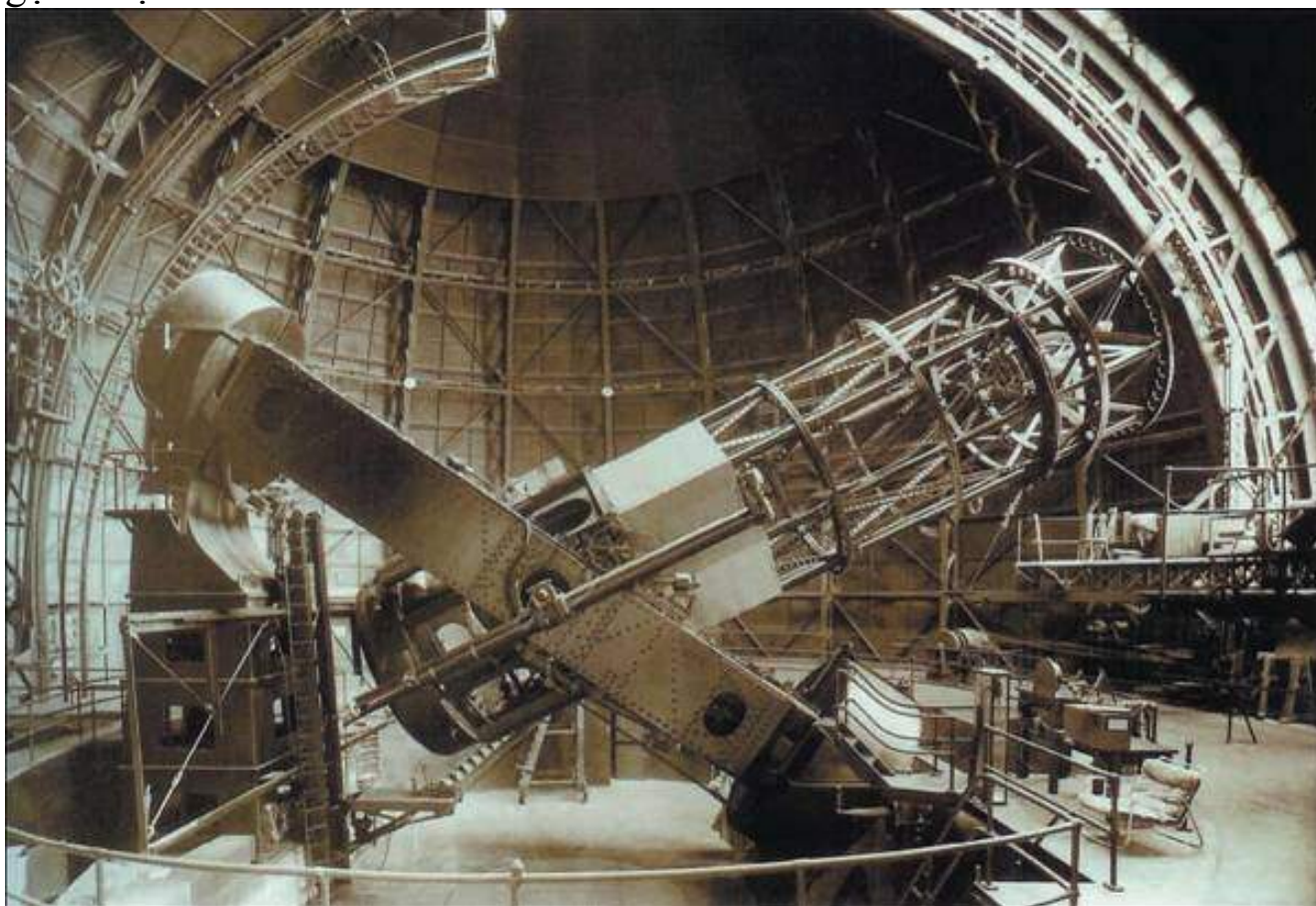
Kính viễn vọng 100-inch tại đài quan sát Mount Wilson.
