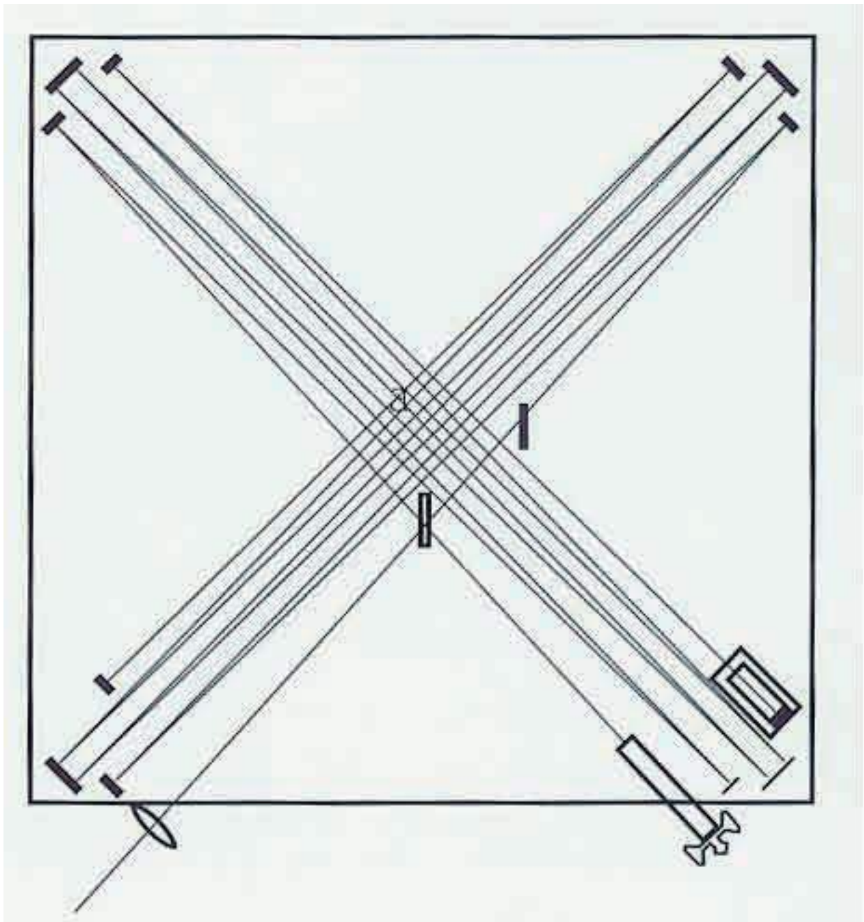
Hình phải: sơ đồ thí nghiệm được vẽ lại từ sơ đồ được in trên tạp chí Scientific American năm 1887.
