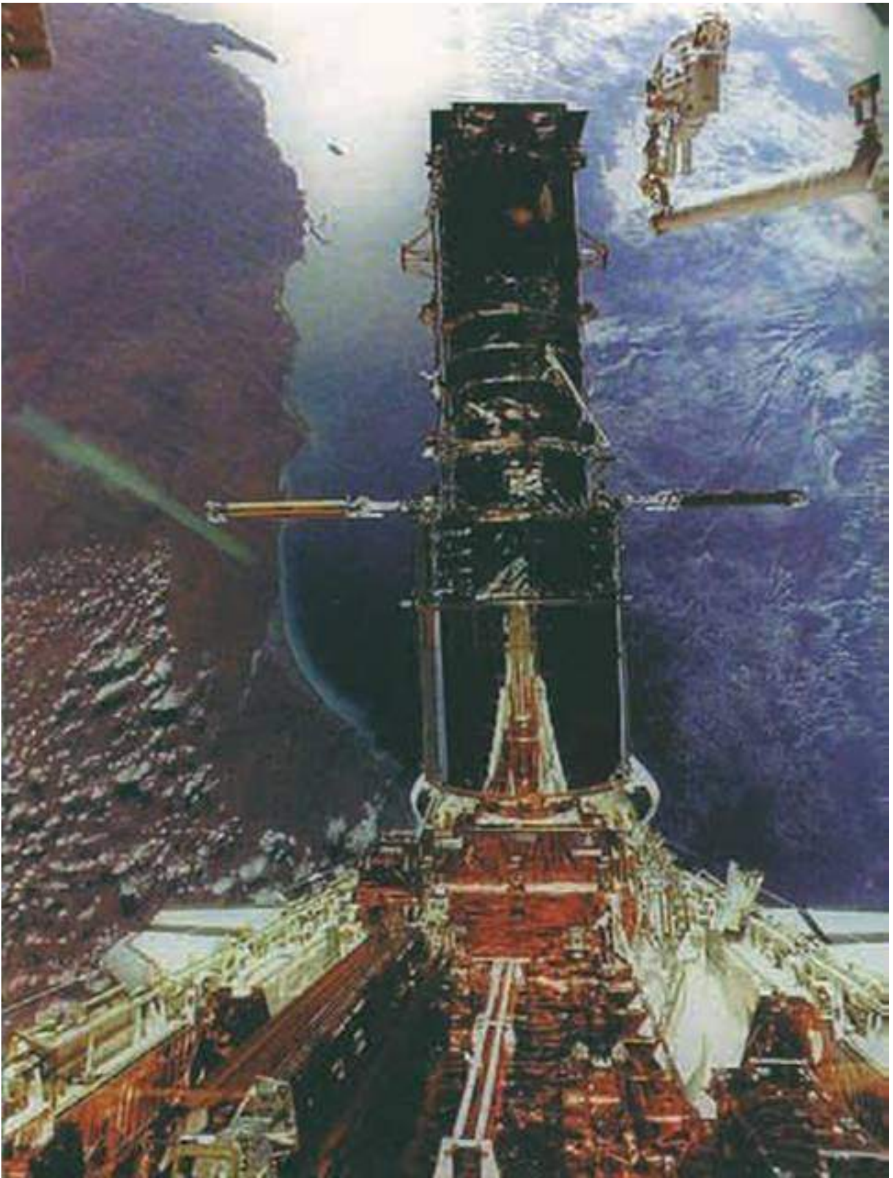
Một phi thuyền con thoi đang nâng cấp ống kính và gương của đài thiên văn vũ trụ Hubble. Phía dưới là lục địa Úc.
