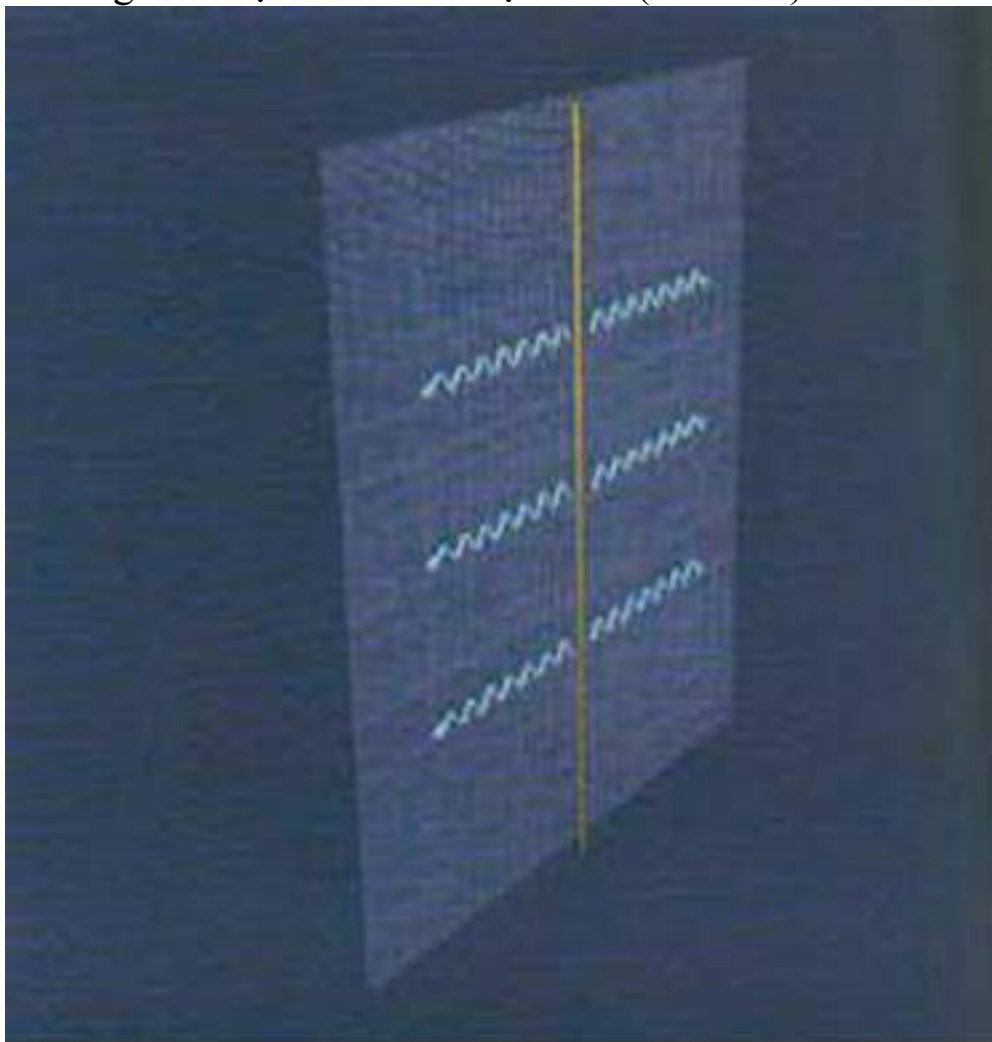
(Hình 7.7) THẾ GIỚI MÀNG
