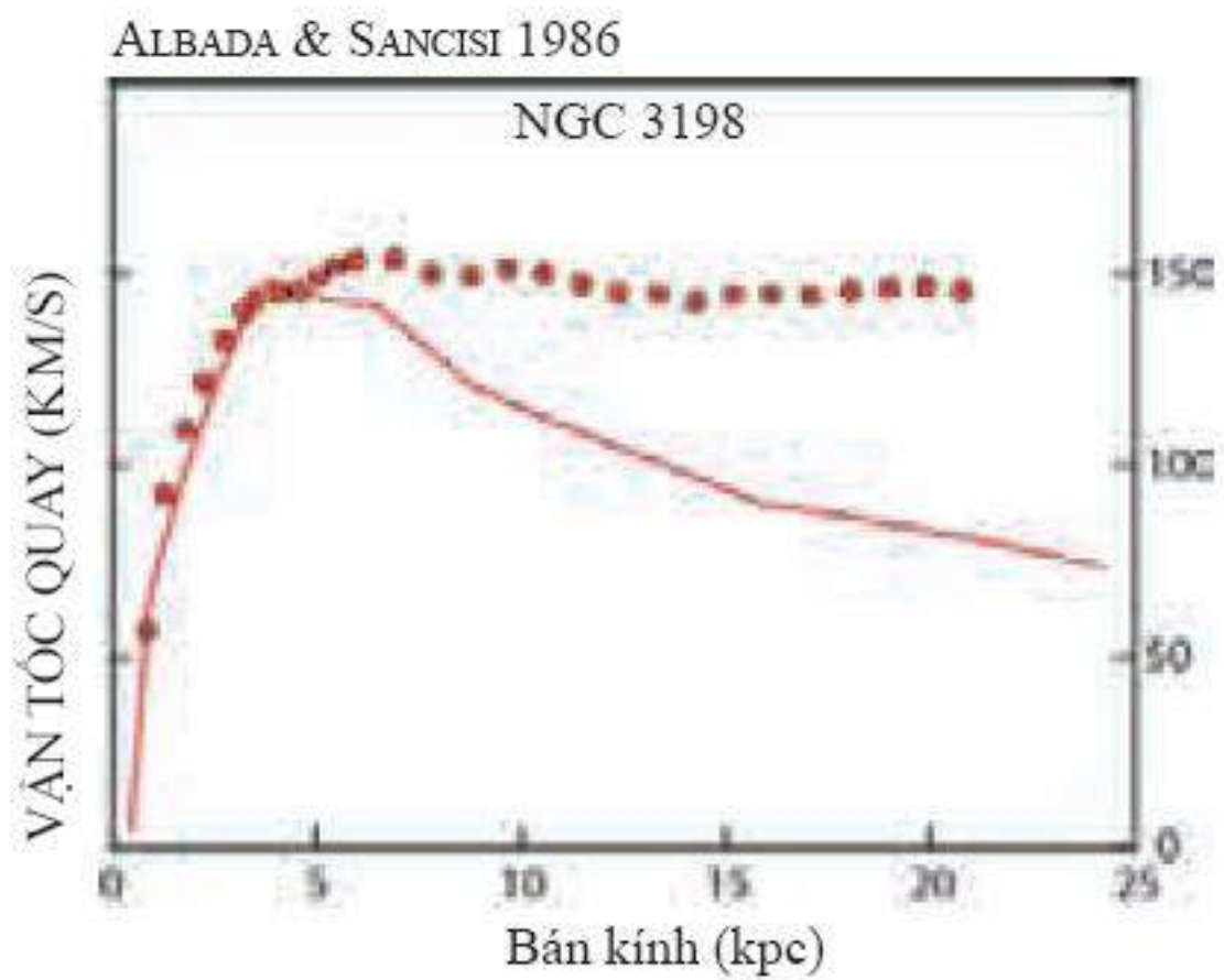
THIÊN HÀ XOÁY ỐC NGC 3198
