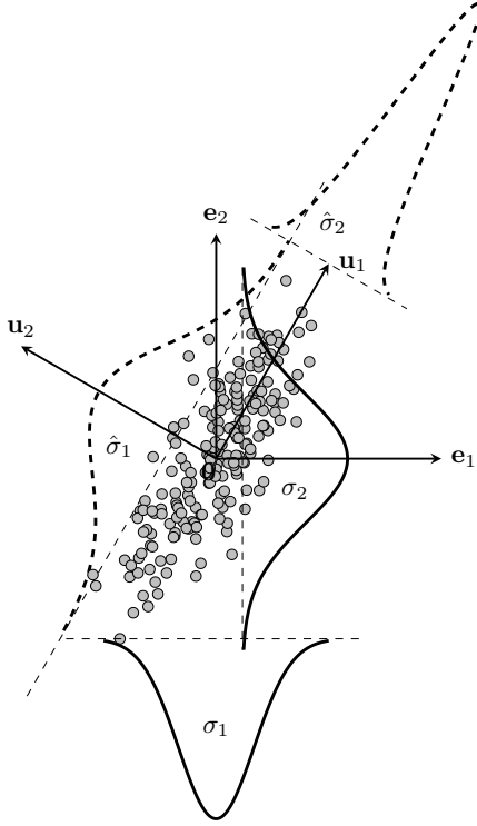
Hình 21.3. PCA có thể được coi là phương pháp đi tìm một hệ cơ sở trực chuẩn đóng vai trò một phép xoay, sao cho trong hệ cơ sở mới này, phương sai theo một số chiều nào đó là không đáng kể và có thể lược bỏ. Trong hệ cơ sở ban đầu \mathbf{Oe}_1\mathbf{e}_2 , phương sai theo mỗi chiều (độ rộng của các đường hình chuông nét liền) đều lớn. Trong không gian mới với hệ cơ sở \mathbf{Ou}_1\mathbf{u}_2 , phương sai theo hai chiều (độ rộng của các đường hình chuông nét đứt) chênh lệch nhau đáng kể. Chiều dữ liệu có phương sai nhỏ có thể được lược bỏ vì dữ liệu theo chiều này ít phân tán.
