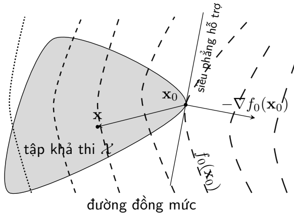
Hình 24.2. Biểu diễn hình học của điều kiện tối ưu cho hàm mục tiêu khả vi. Các đường nét đứt tương ứng với các đường đồng mức. Nét đứt càng gần ứng với giá trị càng cao.
