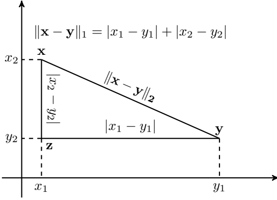
Hình 1.2. Minh họa chuẩn \ell_1 và chuẩn \ell_2 trong không gian hai chiều. Chuẩn \ell_2 chính là khoảng cách Euclid. Trong khi đó chuẩn \ell_1 là quãng đường ngắn nhất giữa hai điểm nếu chỉ được đi theo các đường song song với các trục tọa độ.
