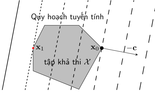
Hình 24.3. Biểu diễn hình học của quy hoạch tuyến tính
