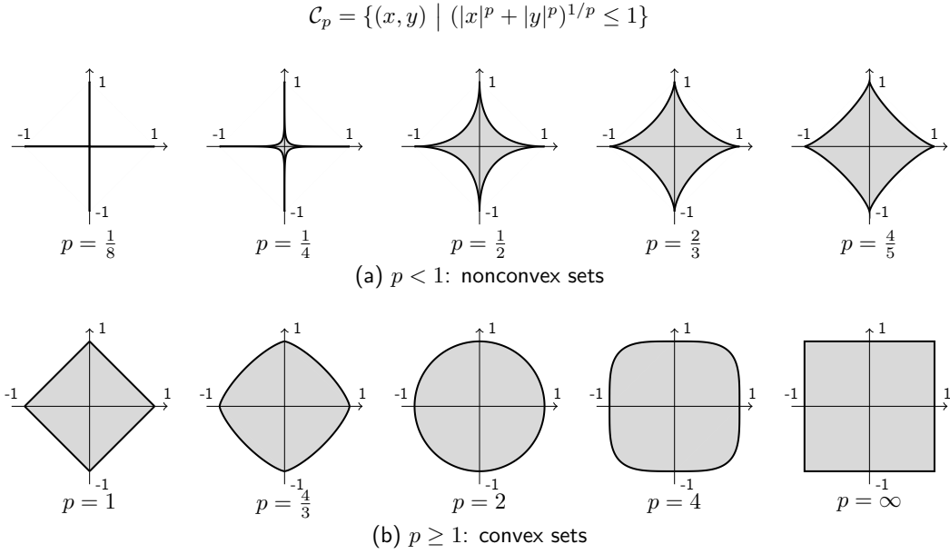
Hình 23.3. Hình dạng của các tập hợp bị chặn bởi các (a) giả chuẩn và (b) chuẩn.
