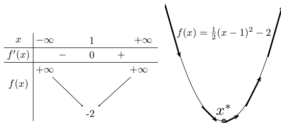
Hình 12.1. Khảo sát sự biến thiên của một đa thức bậc hai.
