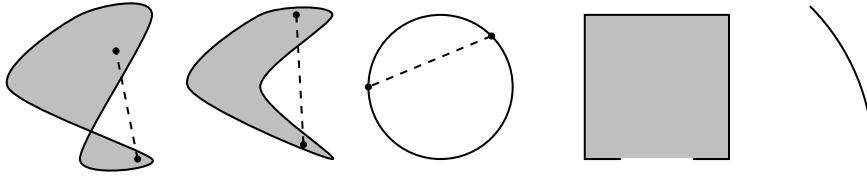
Hình 23.2. Các ví dụ về tập không lồi.
