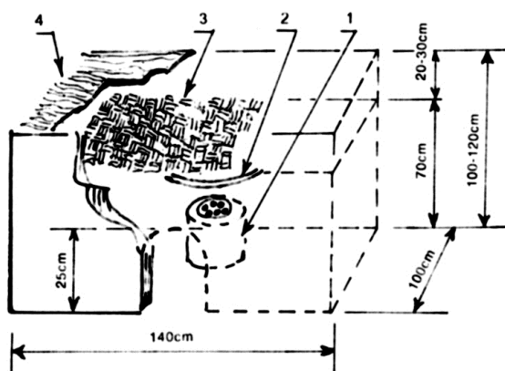
Hình 9: Cấu tạo lò sấy vải
