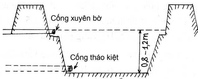
Mặt cắt ao nuôi tôm
