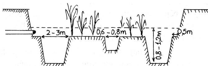
Mặt cắt ruộng nuôi tôm
