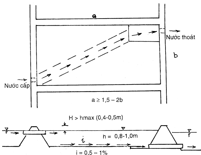
Sơ đồ ao nuôi tôm (Theo Phạm Văn Tình, 1994).
