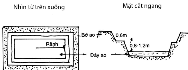
Hình dáng ao nuôi cá trê
