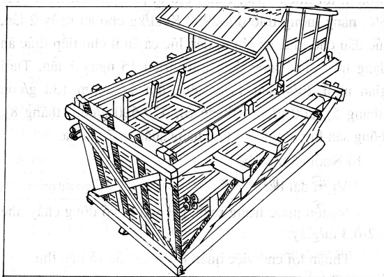
Kết cấu bè nuôi cá tra ở tỉnh Đồng Tháp (1995)
