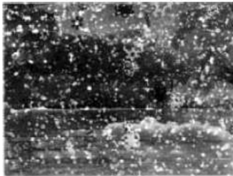
Snowflakes: các bông tuyết rơi
