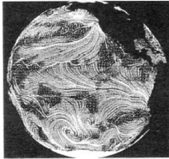
Ocean curenrs Các dòng chảy đại dương
