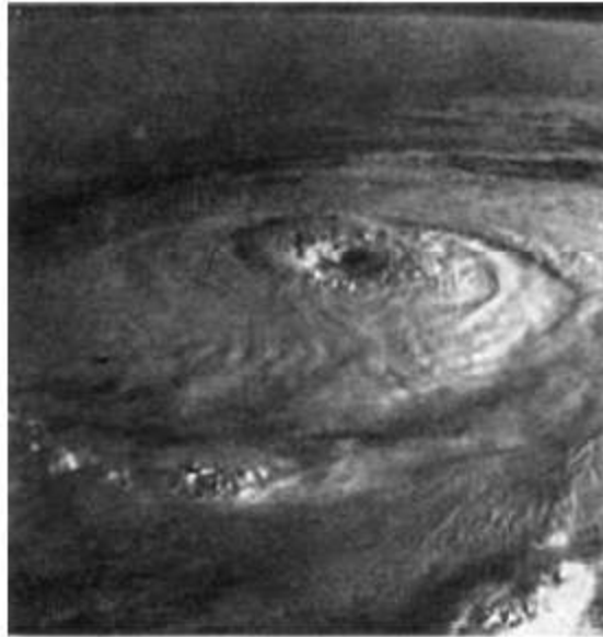
Hurricanes Bão tố
