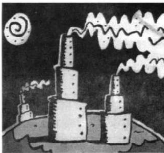
Global warning Hiện tượng trái đất ấm dần lên
