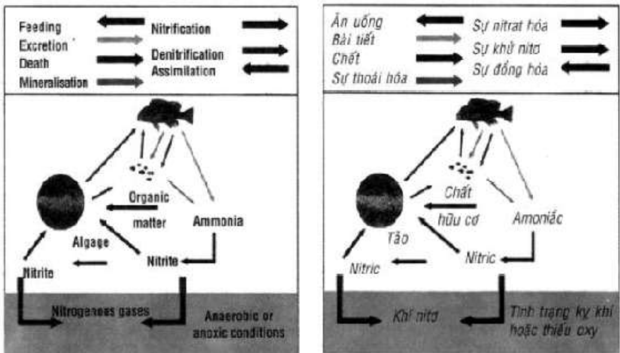
Nitrogen Cycle: chu kỳ Nitơ
