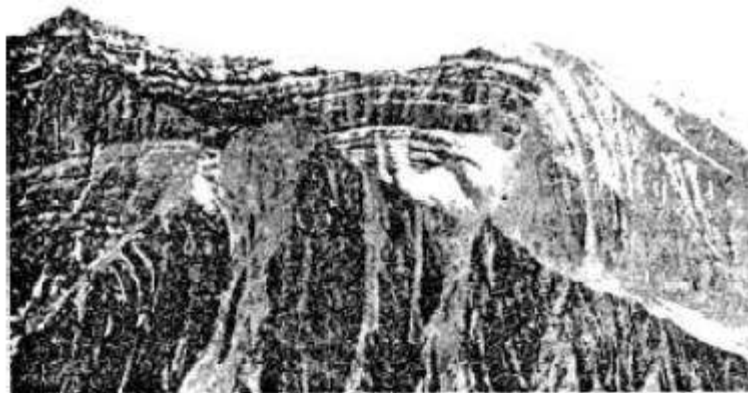
Fold mountain Núi gấp
