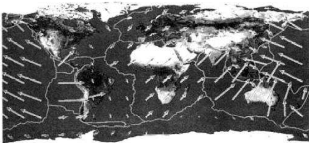
Plate movement Sự di chuyển của phiến lục địa
