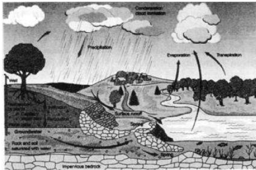
Mechanism of Rainfall Cơ cấu lượng mưa
