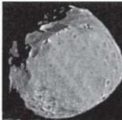
Phobos Vệ tinh Phobos
