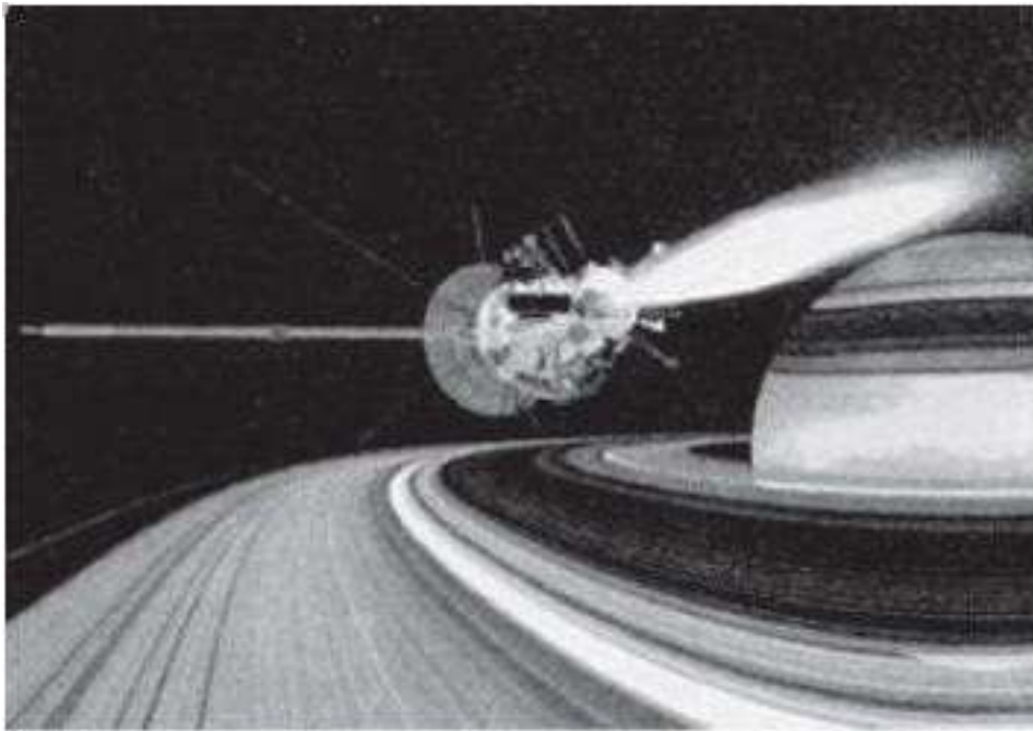
Close view of Staturm's ring Cận ảnh của quầng sao Thổ
