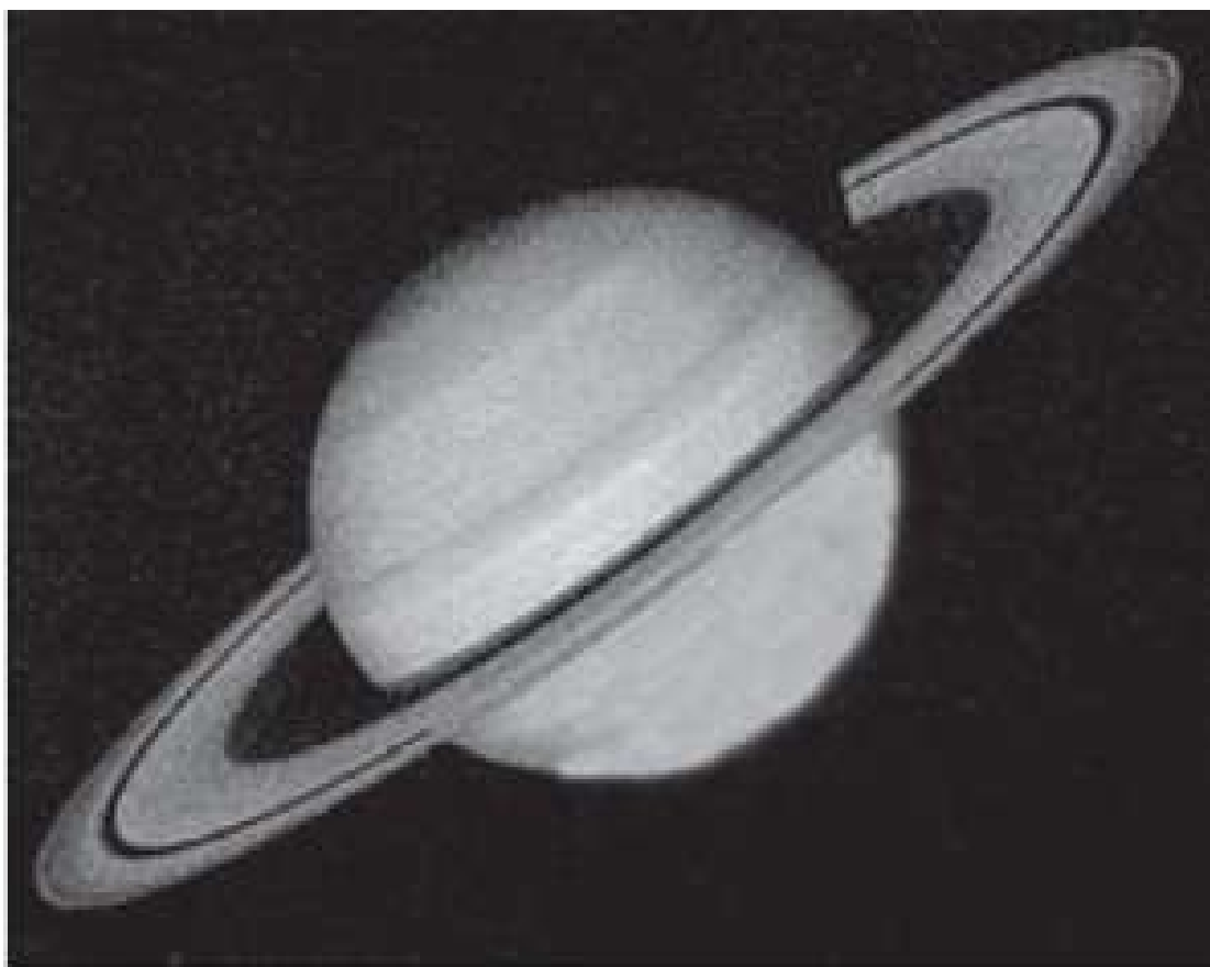
Saturn Sao Thổ
