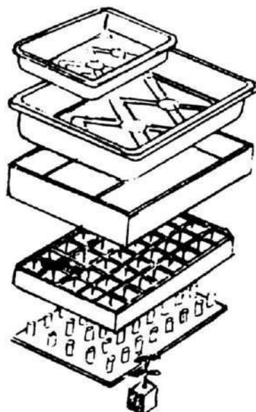
Các loại khay bằng chất dẻo
