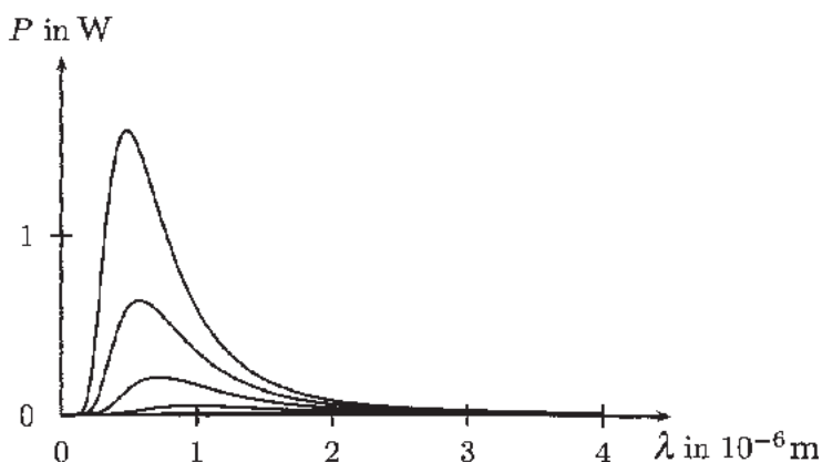
Hình 2.1. Hàm phân bố phổ của vật đen ở những nhiệt độ khác nhau.
