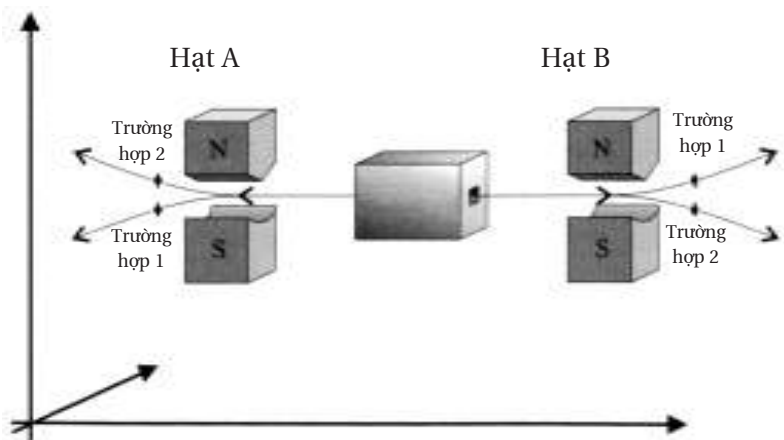
Hình 15.3. Thí nghiệm EPR của Bell theo lý thuyết các biến số ẩn
