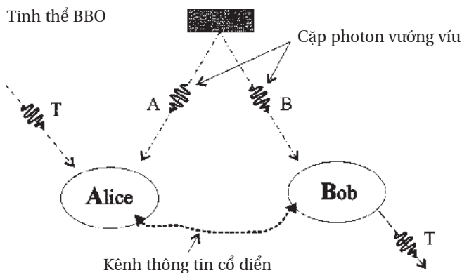
Hình 16.1. Sơ đồ thiết kế thí nghiệm viễn tải lượng tử.
