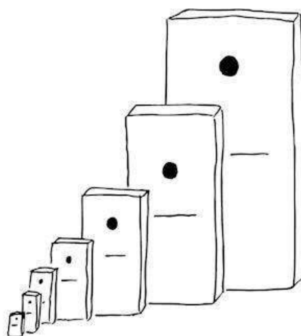
Hình 1: Một dãy chuyển domino cấp số nhân
