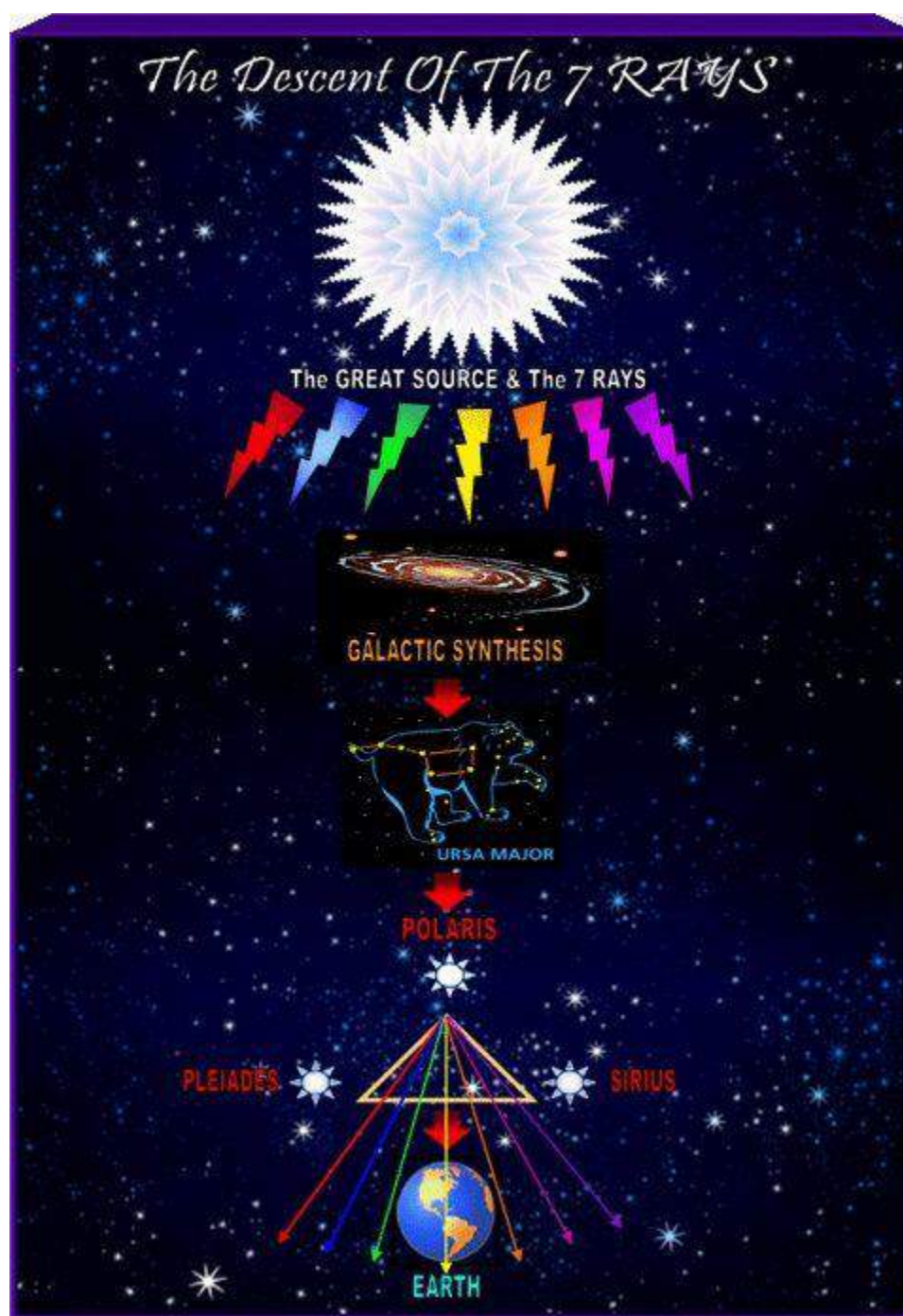
Đường đi của các tia năng lượng tới Trái Đất
