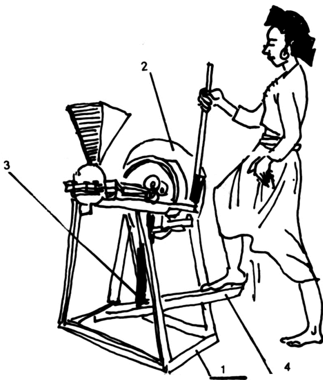
Hình 9: Máy nghiền ngô đạp chân
