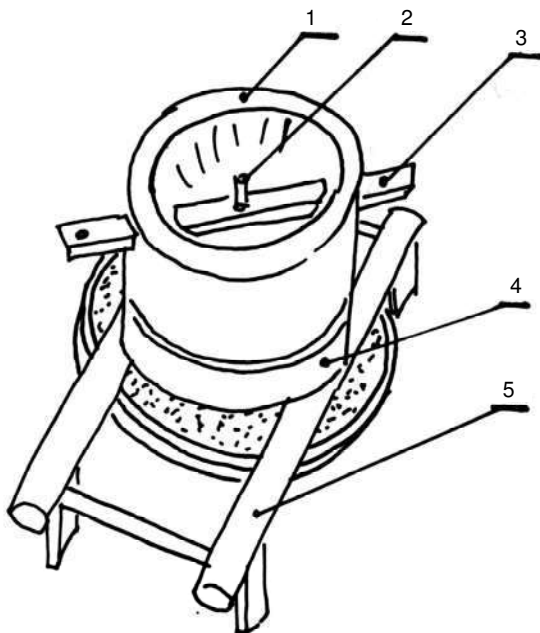
Hình 8: Cối xay ngô
