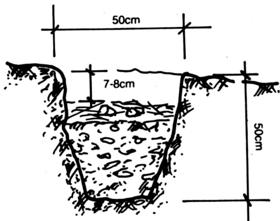
Hình 6: Kích thước hốc
