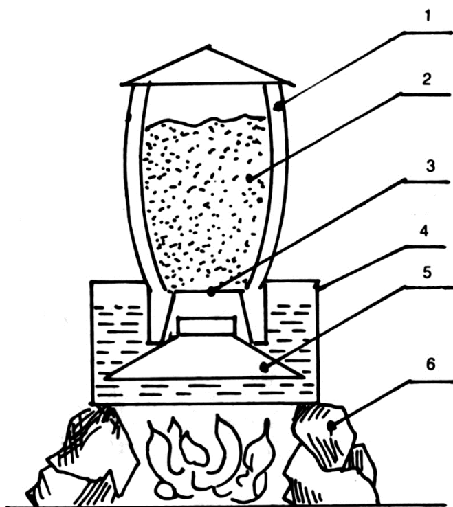
Hình 10: Nồi đất cải tiến đồ ngô
