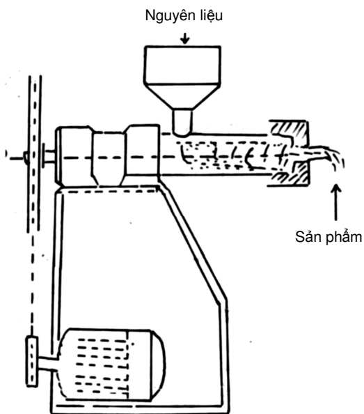
Hình 12: Máy ép đùn
