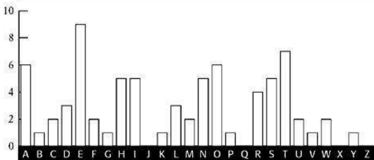
Hình 16. Phân bố theo L_1 được dịch lùi lại bốn chữ cái (hình bên trên) so với phân bố tần suất chuẩn (hình bên dưới). Tất cả các đỉnh và hõm chính
