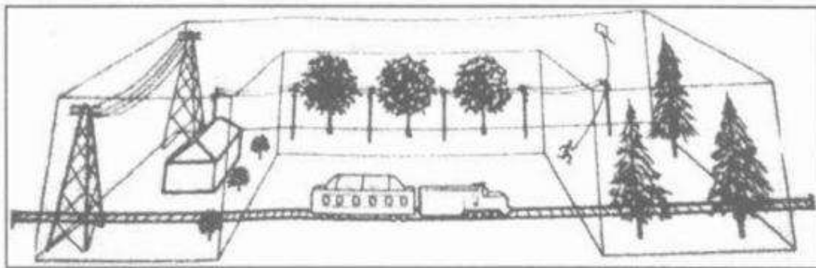
Hình 9.4. Phong cảnh nhìn từ con tàu chuyển động với vận tốc 8 km/h.
