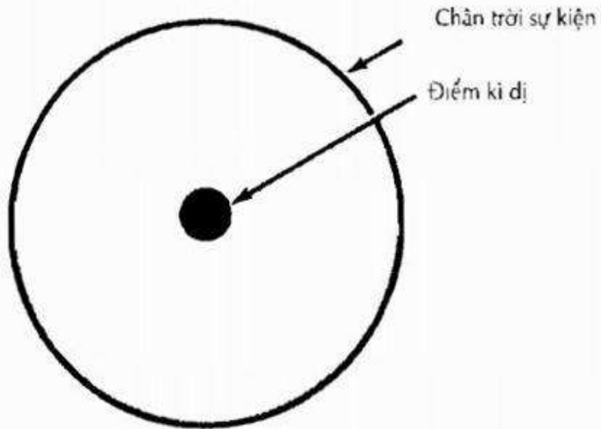
Hình 23.11. Một lỗ đen
