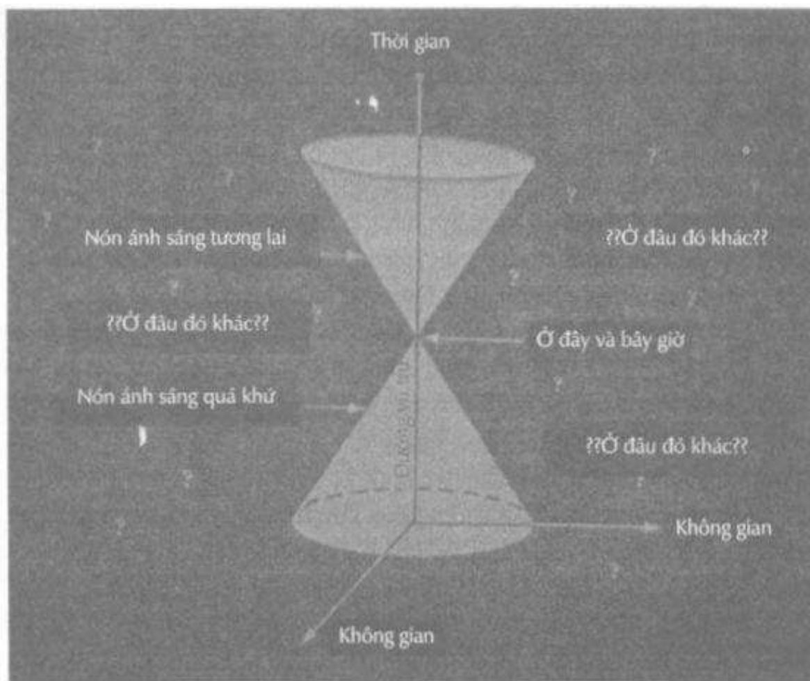
Hình 17.3. Hình nón ánh sáng của không-thời gian.
