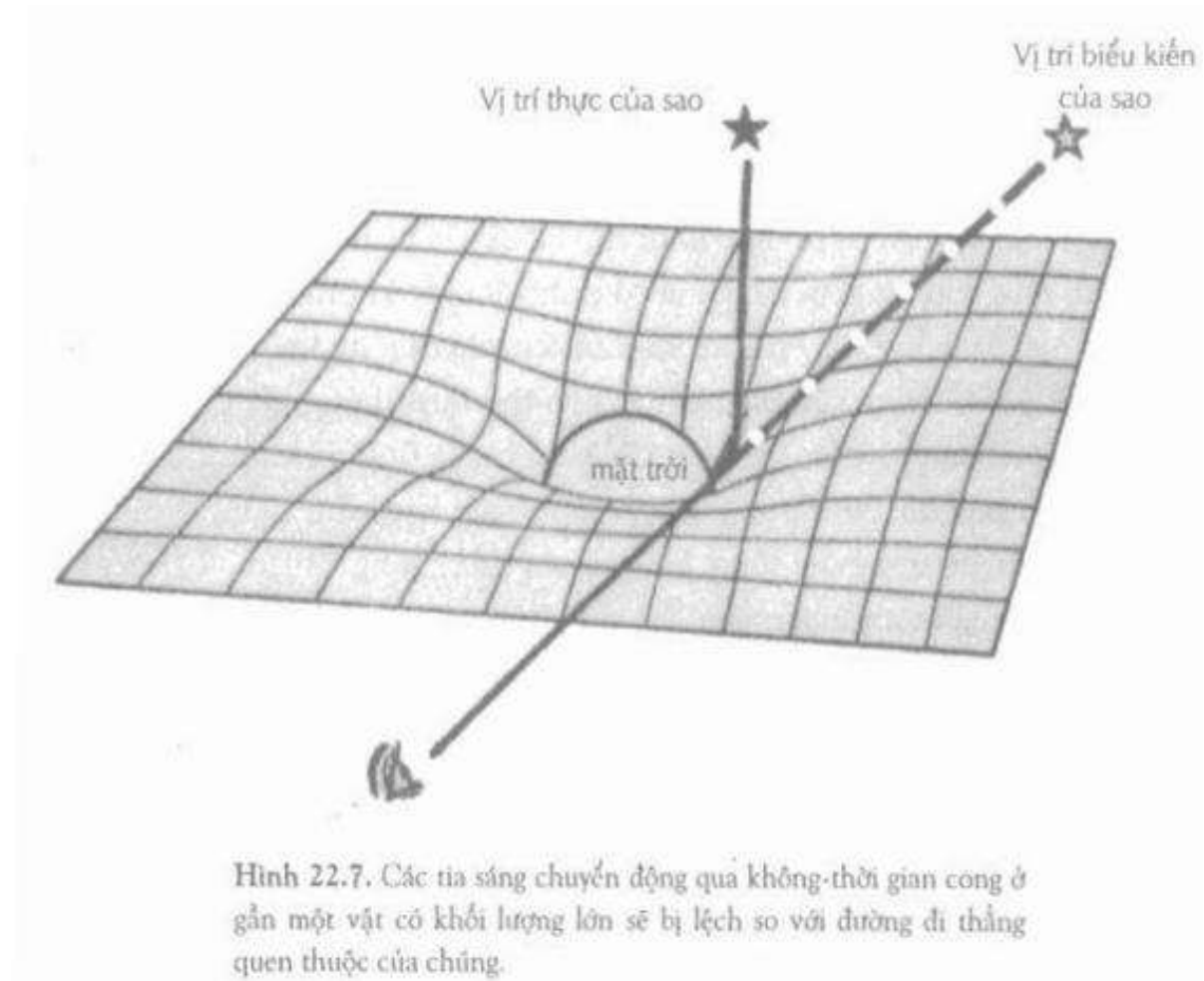
Hình 22.7. Các tia sáng chuyển động qua không-thời gian cong ở gần một vật có khối lượng lớn sẽ bị lệch so với đường đi thẳng quen thuộc của chúng
