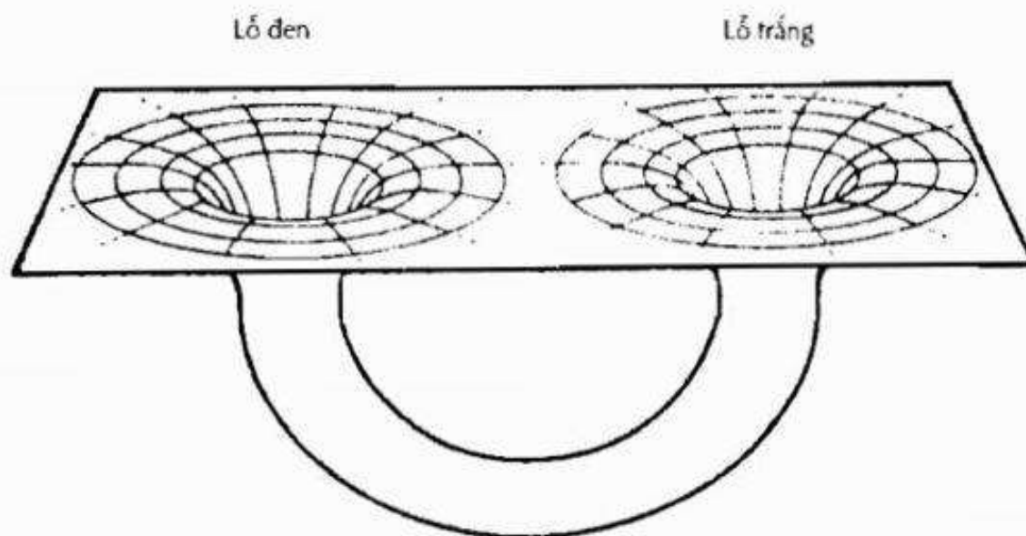
Hình 23.13. Một đường hầm giun đào trong không-thời gian: đầu kia của một lỗ đen trong vũ trụ chúng ta có thể sẽ mở ra ở một vị trí khác tại một thời gian khác.
