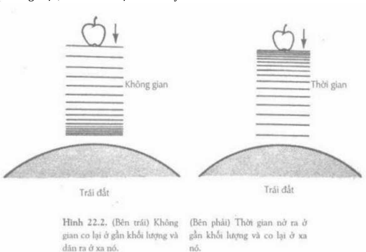
Hình 22.2. (Bên trái) Không (Bên phải) thời gian nở ra ở gian co lại ở gần khối lượng và gần khối lượng và co lại ở xa giãn ra ở xa nó.
