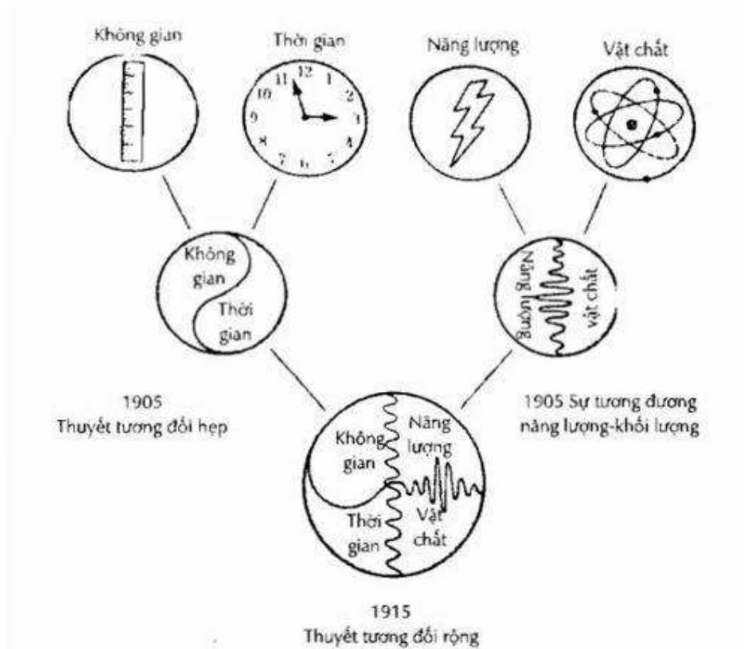
Hình 22.1. Đồ hình của thuyết tương đối rộng
