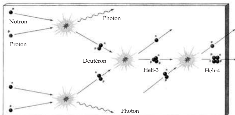
Hình 40. Sự hình thành hêli-4 trong vũ trụ nguyên thủy. Một proton và một notron kết hợp với nhau để tạo thành một deuteron (đơteron) kèm theo sự giải phóng năng lượng dưới dạng một photon. Đơteron này lại kết hợp với một proton để tạo thành một hạt nhân hêli-3. Hạt nhân này sau đó kết hợp với một notron để tạo thành một hạt nhân hêli-4 (hêli thông thường). Hạt nhân hêli này được cấu thành từ hai proton và hai notron.
