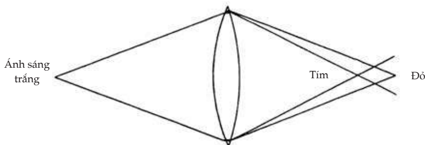
Hình 18. Sắc sai . Các mép của một thấu kính trong kính thiên văn khúc xạ xử sự như một lăng kính và làm lệch các thành phần màu theo các góc khác nhau. Chẳng hạn, thành phần tím bị lệch nhiều hơn và tụ tiêu tại một điểm gần thấu kính hơn thành phần đỏ. Điều này có nghĩa là tất cả hình ảnh thu được về các thiên thể đều có một quang màu, dù vị trí của máy dò được đặt ở đâu giữa các tiêu điểm các ánh sáng tím và đỏ.
